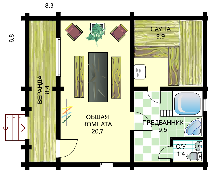
М 1:100
